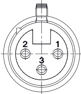
Abb. 13: Batterieanschluss, Buchse
