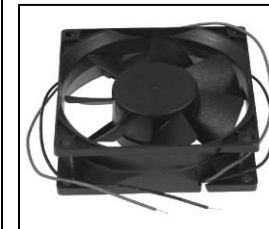
L4.83497.E Fan 12 V / 0,25 A Lüfter 12 V / 0,25 A
