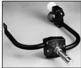
L4.83137.E Stirrup p.o. Haltebügel p.o. further p.o.-spare-parts on sperate sheet weitere p.o. Ersatzteile auf separatem Blatt
