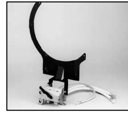
L4.82225.E Lampholder + lamp carriage compl. 100-120 V Lampenfassung + Fassungsträger kpl. 100-120 V L4.82226.E 200-240 V
