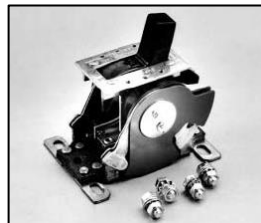
L4.83055.E Switch On/Off 200.240 V Schalter Ein/Aus 200.240 V
