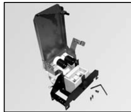
L4.80751.E Lamp holder & carriage for rear loader versions Lampenfassung & Fokusschlitten für Hecklader Version
