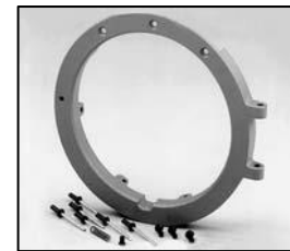
L4.73786.E to ser. no. 1758 / bis Ser. Nr. 1758 Front casting / Frontteil
