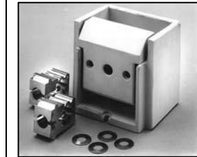
L4.73533.E Lamp holder complete Lampenfassung komplett
