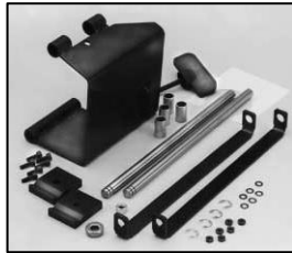
L4.83285.E Justable stirrup bracket set right Schwerpunktverstellung rechts
