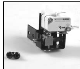
L4.77395SE Safety switch H.T. complete / Endschalter H.T. komplett
