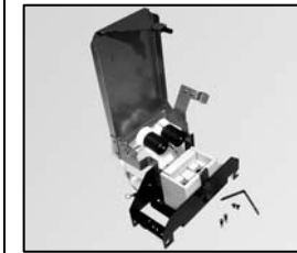
L4.74040.E Lampholder + lamp carriage Lampenfassung + Fokusschlitten
