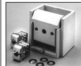
L4.73533.E Lampholder complete Lampenfassung komplett
