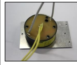
L4.90390.E Ab ser. 6729/from ser. 6729 Ignitor/ Zündgerät
