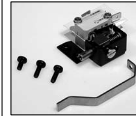
L4.79837.E Safety switch cpl. Endschalter kpl.
