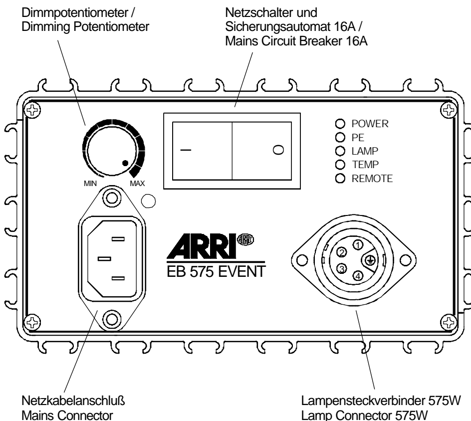
Abb./Fig. 2: Bedienelemente auf der Frontplatte Operating Parts on Front Panel
