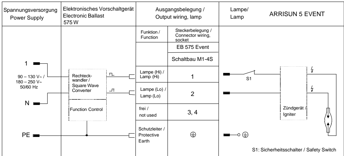
Abb./Fig. 1: Anschlußbelegung 575 W / Connector Wiring 575 W
