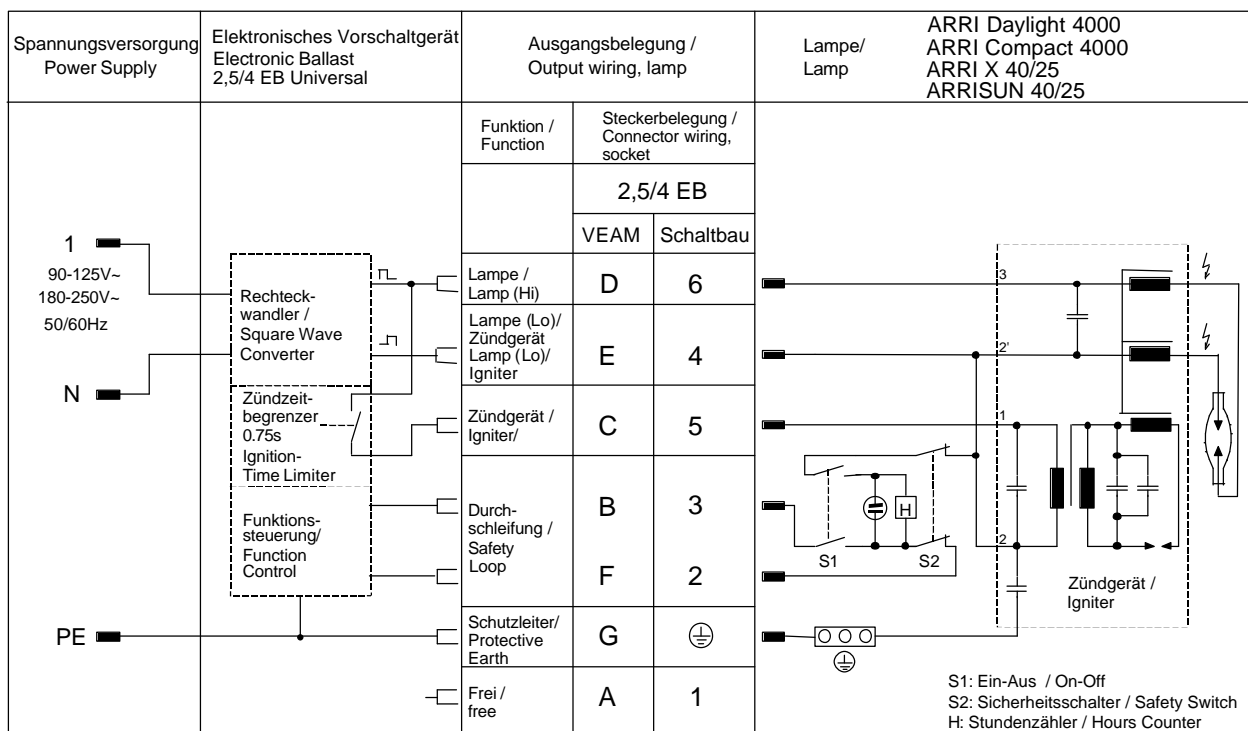
Abb./Fig. 1b: Anschlußbelegung 4000 W / Connector Wiring 4000 W
