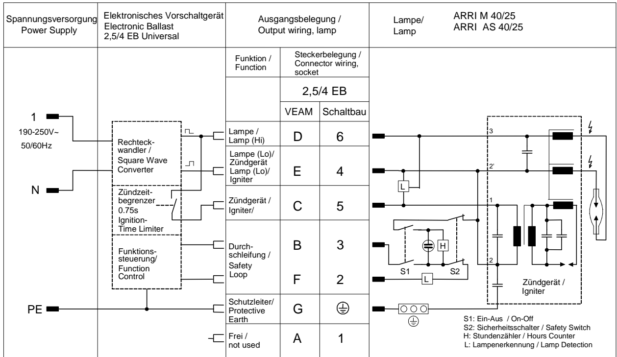
Abb./Fig. 1c: Anschlußbelegung 4000 W mit CCL / Connector Wiring 4000 W with CCL
